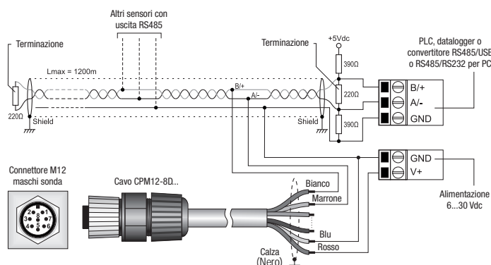
Fig. 4: collegamento RS485
