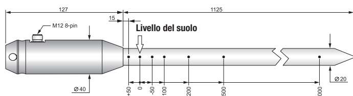
Fig. 1: dimensioni della sonda TP32MTT.03 (mm)
